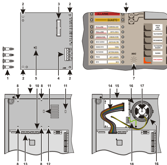
Figura 1 Identificazione delle Parti e Installazione del Modulo Telecom- Schema di collegamento Linea di Riserva
